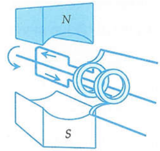
Khung dây quay quanh từ trường đều
